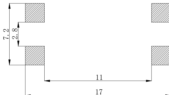
焊接尺寸图
